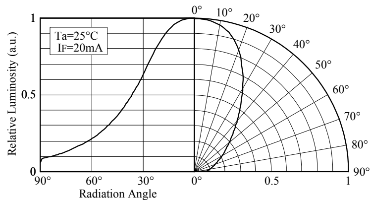
■ Directivity (NSPW515B(S))
